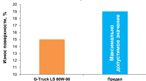
Износ поверхности конической шестерни гипоидной передачи*
